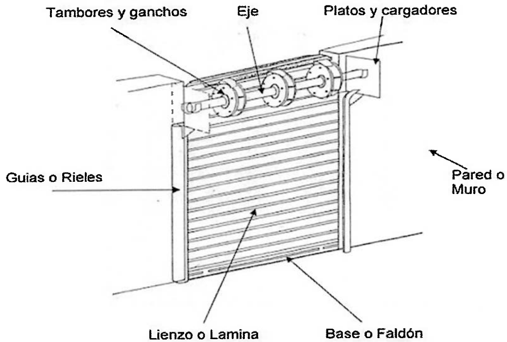
Fig. 3: Muestra esquema de partes elementos principales que componen el sistema cortina enrollable instalada, Ref.: imagen propia.
